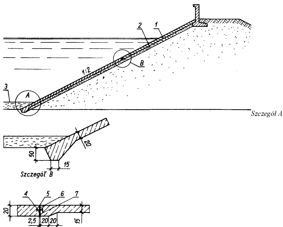
Rys. 7.2. Ekrany żelbetonowe skarpy odwodnej. 1 - płyty betonowe zbrojone w osi siatką z prętów \varnothing 10 co 25 cm, 2 - podsypka żwirowa grub. 30 cm, 3 - fartuch z gliny, 4 - taśma PCW, 5 - korek betonowy, 6 - masa zalewowa, 7 - deska
