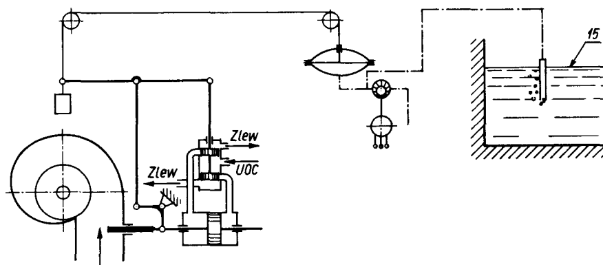
Rys. 9.6. Regulator mocy z czujnikiem pneumatycznym i siłownikiem membranowym
