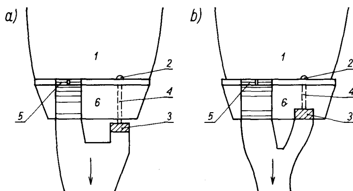
Rys. 6.5 Usytuowanie elektrowni przy zaporach betonowych: a) układ klasyczny, b) układ z elektrownią w sekcji zapory, 1 - zbiornik, 2 - ujęcie wody, 3 - elektrownia, 4 - rurociąg, 5 - przelew, 6 - zapora
