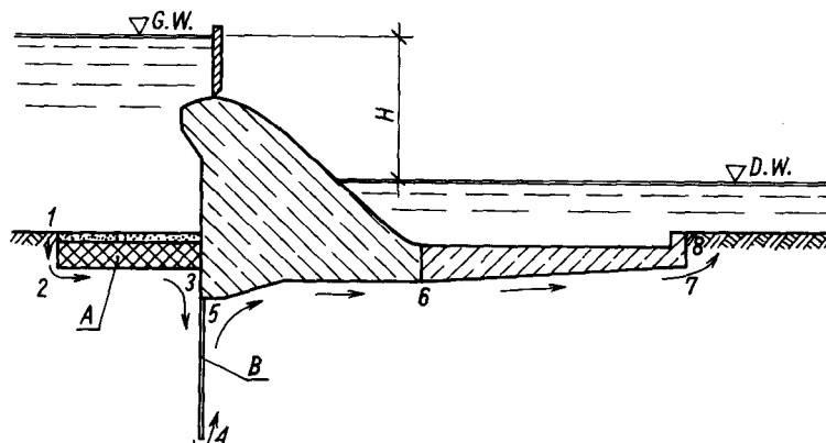
Rys. 7.6. Droga filtracji pod jazem. A – fartuch iłowy, B – ścianka szczelna
