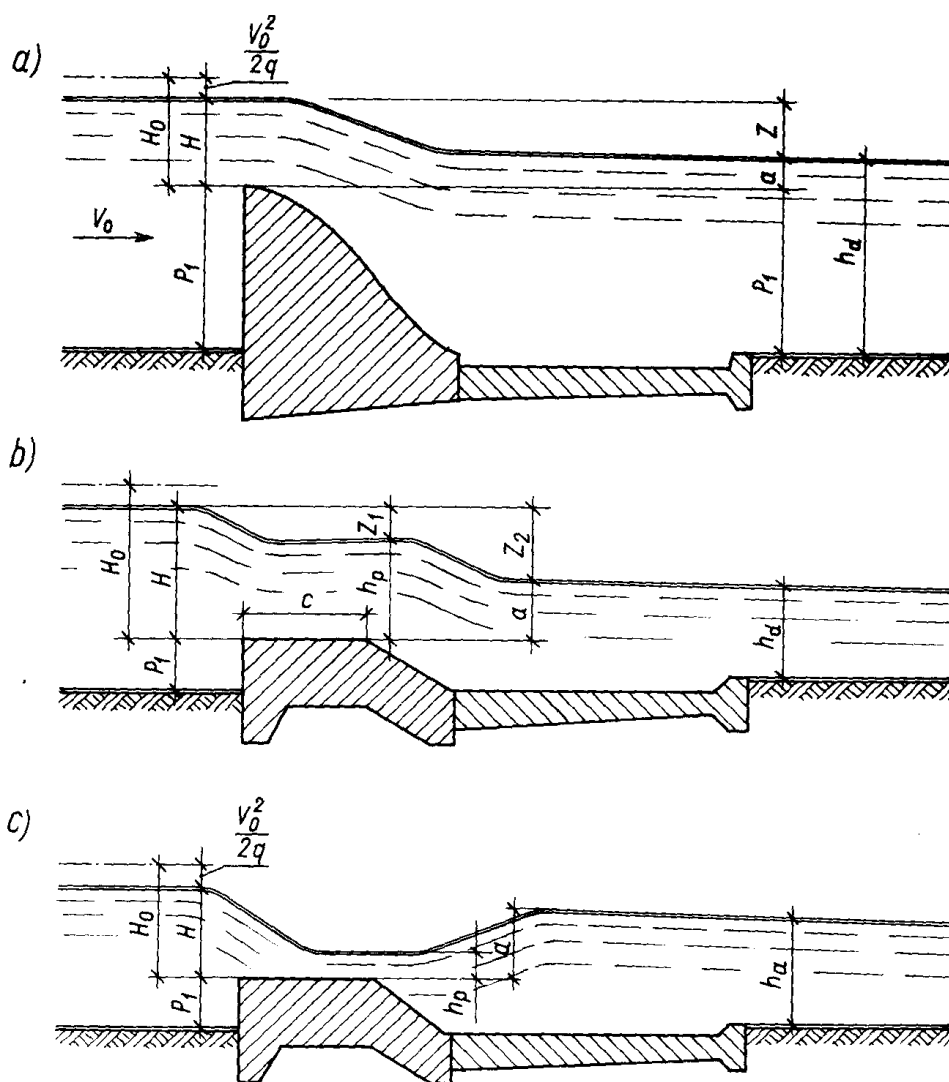
Rys. 7.7. Rodzaje przelewów: a) o kształtach praktycznych, b) o szerokiej koronie niezatopiony ( a \ll h_p ), c) o szerokiej koronie zatopiony
