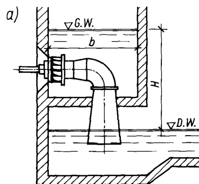
Rys. 7.17. Rura ssąca: a) z kolaniem zanurzonym w wodzie, b) z kolaniem suchym
