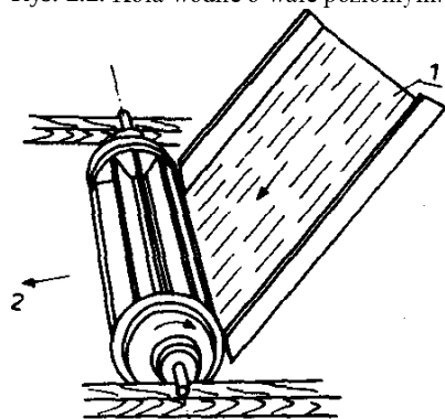
Rys. 2.3. Koło wodne „Walaska”. 1 - rynna doprowadzająca wodę, 2 - odprowadzenie wody
