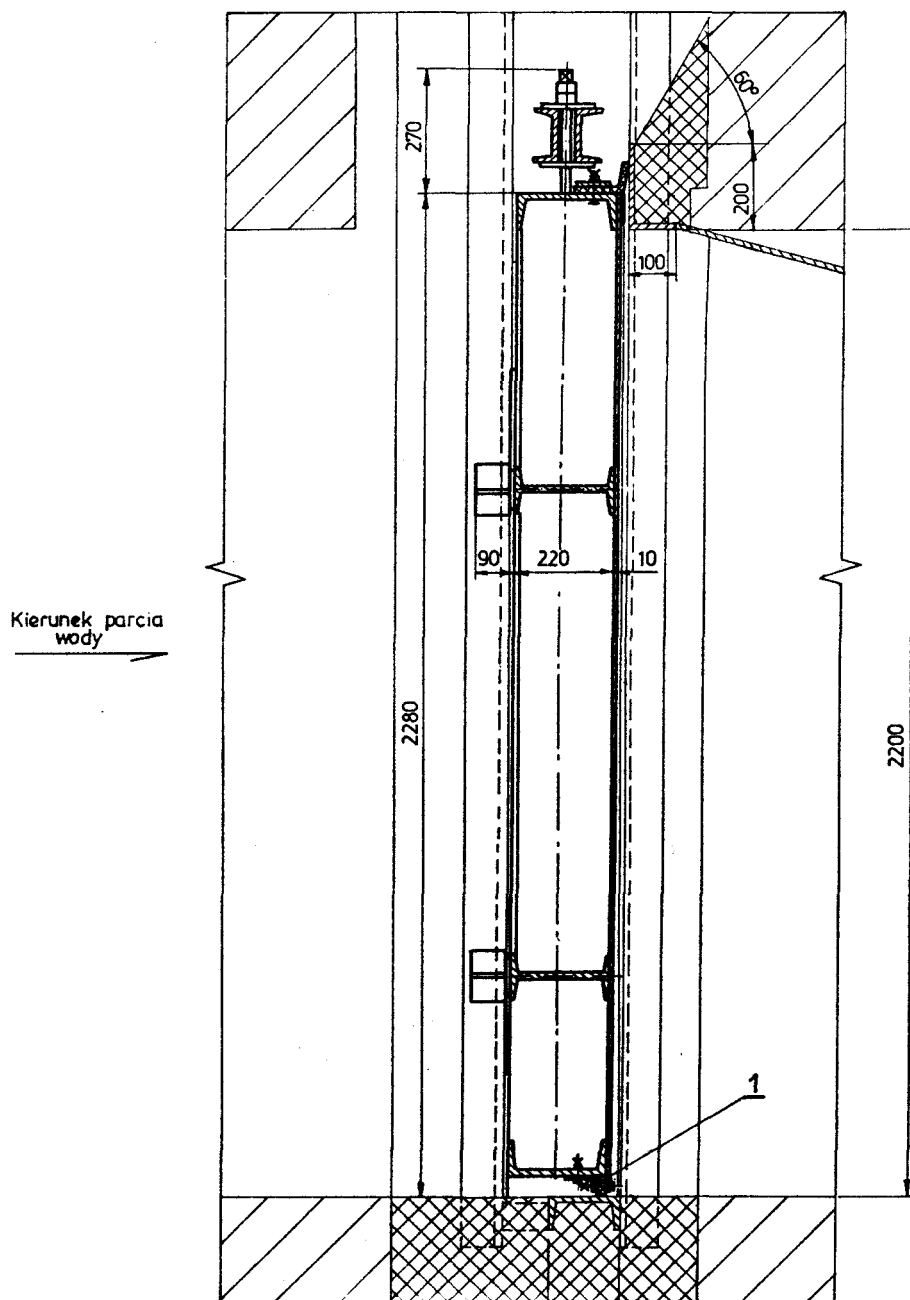
Rys. 12.5. Zastawka stalowa. 1 – uszczelnienia gumowe
