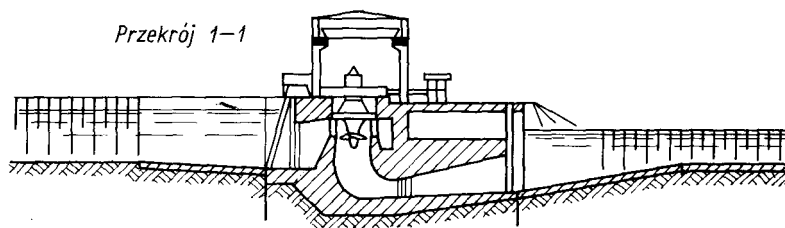
Rys. 6.1. Elektrownia przyjazowa. 1 - śluza, 2 - jaz, 3 - elektrownia
