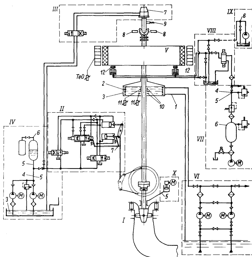
Rys. 9.8. Schemat hydromechaniczny turbozespolu. I - turbina Kaplana, II - ser-womotor aparatu kierowniczego, III - ser-womotor nastawiania lopat wirnika, IV - stacja zasilania hydraulicznego, V - prądnica synchroniczna, VI - pompy wody chłodzącej łożysko prądnicy, VII - urządzenia sprężarkowe, VIII - stanowisko hamowania i podnoszenia zespołu wirującego, IX - przenośny olejowy agregat pompowy
