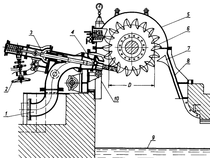
Rys. 8.17. Turbina Peltona. 1 - rurociąg doprowadzający, 2 - sterowanie ręczne, 3 - urządzenie przesuwające iglicę, 4 - dysza z iglicą, 5 - osłona wirnika, 6 - wirnik turbiny,
