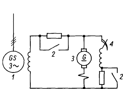
Rys. 11.3. Układ wzbudzenia ze wzbudnicą i ręczną regulacją napięcia. 1 – prądnica, 2 – wyłącznik wzbudzenia, 3 – wzbudnica, 4 – ręczna regulacja napięcia
