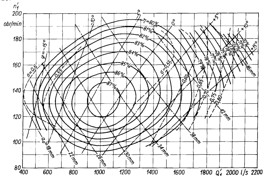
Rys. 8.3. Charakterystyka uniwersalna. \eta – sprawność turbiny \sigma – współczynnik kawitacji, a_0 – otwarcie kierownicy. \varphi kąt ustawienia łopatek wirnika
