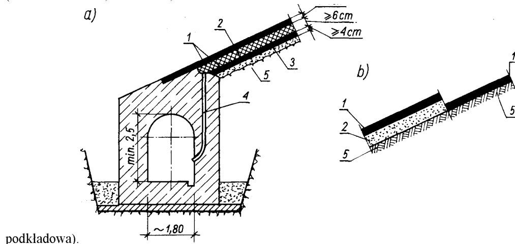
Rys. 7.3. Ekrany asfaltobetonowe: a) ekran dwuwarstwowy, b) ekran jednowarstwowy. 1 - warstwy szczelne ekranu, 2 - warstwa drenażowa, 3 - warstwa wyrównawcza, 4 - odprowadzenie wody, 5 - podłoże
