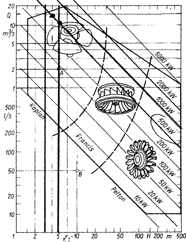
Rys. 8.21. Przykład doboru turbin Kaplana, Francisa, Peltona
