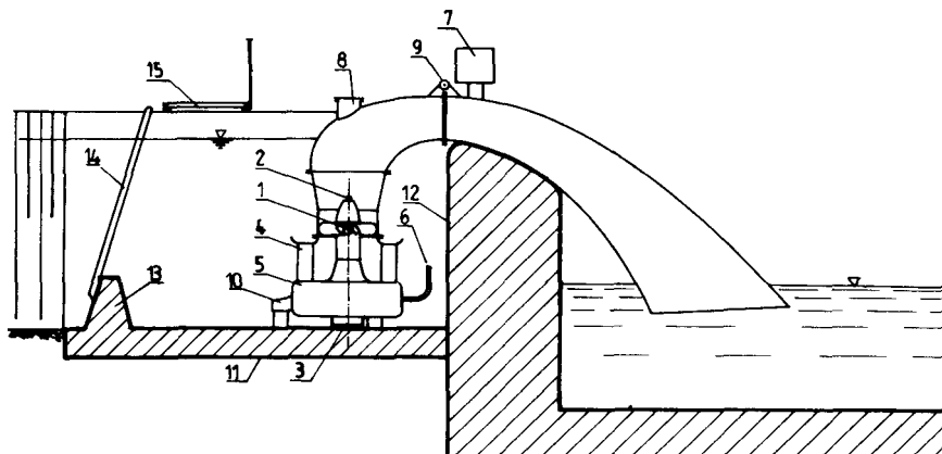
Rys. 15.13. Mała elektrownia wodna z turbozespołem zblokowanym. 1 - wirnik turbiny z łopatkami przestawianymi ręcznie lub automatycznie, 2 - śruba ręcznej regulacji łopatek wirnika, 3 - mechanizm automatycznej regulacji łopatek wirnika (alternatywnie), 4 - stałe łopatki kierownicy, 5 - prądnica, 6 - wyprowadzenie mocy, 7 - agregat odpowietrzający rurę ssącą i awaryjny zawór powietrzny, 8 - luk do śruby regulacyjnej, 9 - zawias, 10 - elementy wsporcze turbozespołu, 11 - płyta fundamentowa turbozespołu, 12 - próg jazu, 13 - próg przeciwrumowiskowy, 14 - kraty wlotowe, 15 - kładka robocza
