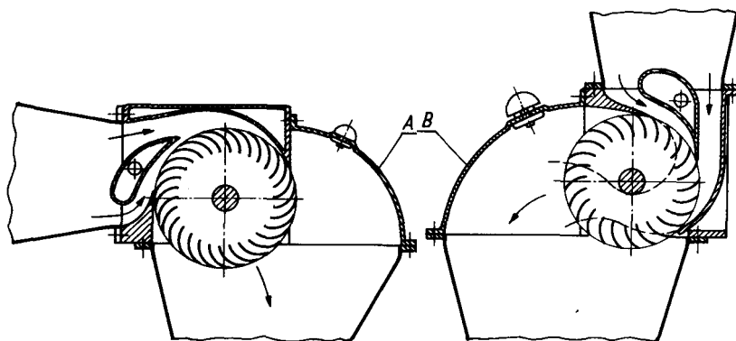
Rys. 8.18. Turbina Banki-Michella - rozwiązania konstrukcyjne. A - poziome doprowadzenie wody, B- pionowe doprowadzenie wody, 1 - korpus turbiny, 2- kierownica, 3 - wirnik, 4 - łożyskowanie wirnika, 5 - osłona wirnika, 6 - zawór napowietrzający, 7 - rura ssąca, 8 - króciec wlotowy
