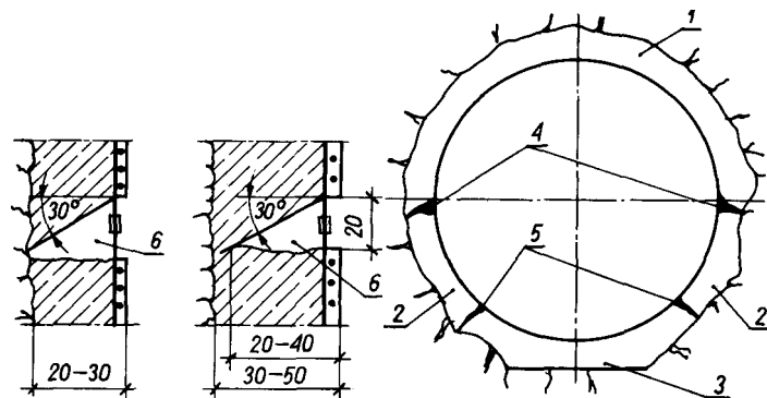
Rys. 7.14. Typowa obudowa betonowa sztolni ciśnieniowej, 1 - szwy robocze, 2 - otwory iniekcyjne
