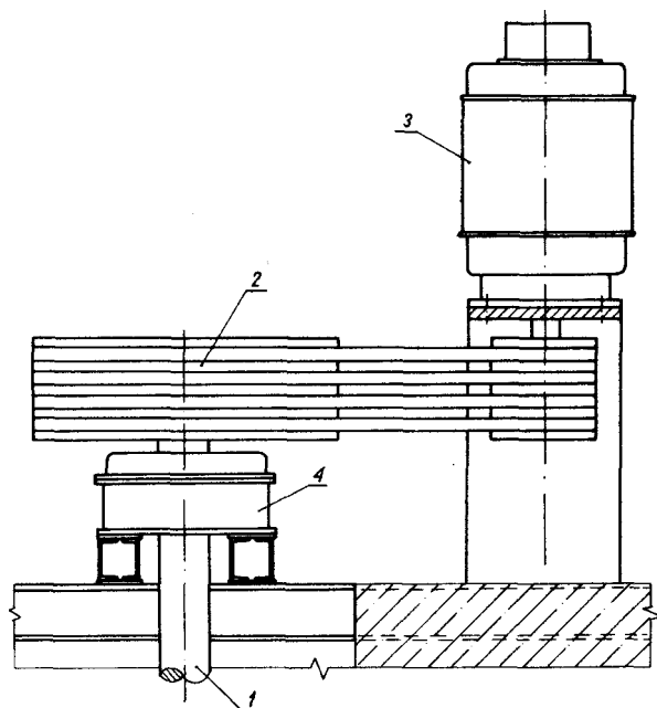
Rys. 10.7. Przekazanie napędu z turbiny na prądnicę za pomocą przekładni z pasami klinowymi w układzie pionowym wałów turbiny i prądnicy, 1 - wał turbiny, 2 - przekładnia, 3 – prądnica
