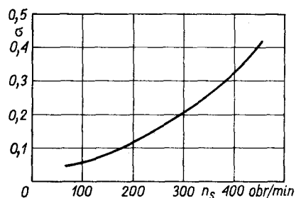
Rys. 8.7. Wartość współczynnika kawitacji \sigma w funkcji wyróżnika szybkobieżności n_s dla turbin Francis
