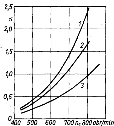
Rys. 8.8. Wartość współczynnika kawitacji \sigma w funkcji wyróżnika szybkobieżności n_s dla turbin Kaplana. 1 – średnio dla starych typów, 2 – średnio dla nowych typów, 3 – wykonania specjalne
