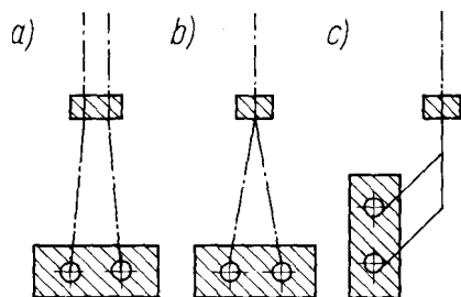
Rys. 6.3. Doprowadzania rurowodów do turbin: a) czołowe indywidualne, b) z rozgałęzieniem, c) boczne z rozgałęzieniem
