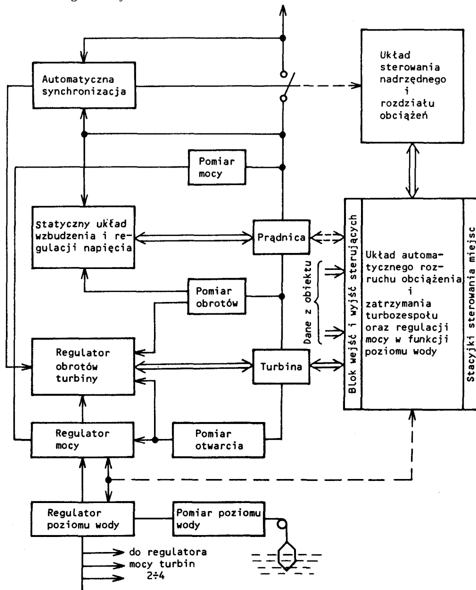
Rys. 14.1. Schemat blokowy układu automatycznego sterowania i regulacji mocy w funkcji poziomu wody MEW z prądnicami asynchronicznymi
