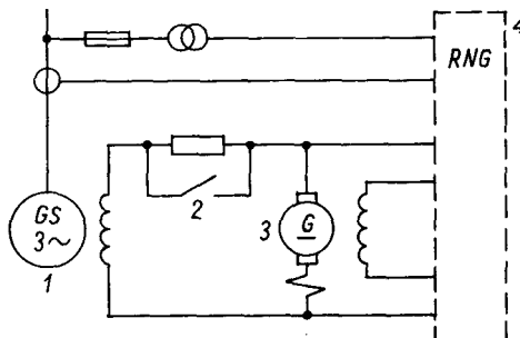
Rys. 11.4. Układ wzbudzenia ze wzbudnicą i automatyczną regulacją napięcia. 1 – prądnica, 2 – wyłącznik wzbudzenia, 3 – wzbudnica, 4 – automatyczny regulator napięcia
