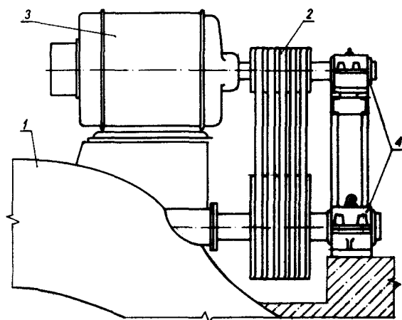
Rys. 10.6. Przekazanie napędu z turbiny na prądnicę za pomocą przekładni z pasami klinowymi w układzie poziomym wałów turbiny i prądnicy, 1 - turbiny rurowa, 2 - przekładnia, 3 - prądnica, 4 - łożyska
