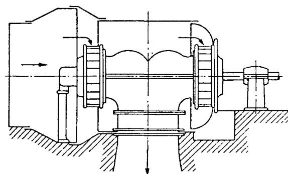
Rys. 8.13. Turbina Francisa z wałem poziomym: a) Francis z krzywkiem, b) Francis w spirali, c) Francis bliźniaczy w kotle
