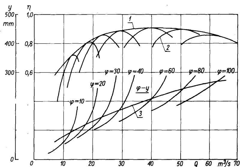
Rys. 8.5. Charakterystyka sprawnościowa turbiny Kaplana. \eta = f(Q) , (1) i jej charakterystyki śmigłowe (2) oraz optymalna zależność kombinatorska \phi - y (3) \phi - otwarcie wirnika, y - skok siłownika kierownicy
