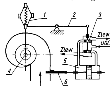
Rys. 9.1. Regulator obrotów mechaniczno-hydrauliczny. 1 - wahadło odśrodkowe, 2 - dźwignia, 3 - suwak rozdzielacza oleju, 4 - turbina, 5 - siłownik kierownicy, 6 - zasawa lub kierownica, UOC - układ olejowo-ciśnieniowy
