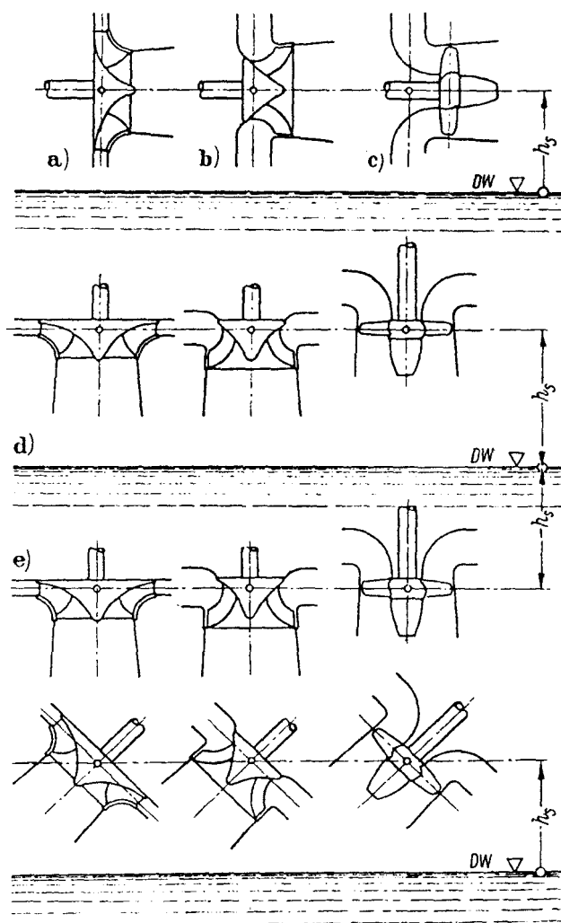
Rys. 8.9. Wysokość ssania h_y a) turbina Francisza wolnobieżna, b) turbina Francisza szybkobieżna, c) turbina Kapłana lub śmigłowa, d) dodatnia wysokość ssania, e) ujemna wysokość ssania, DW- poziom dolnej wody
