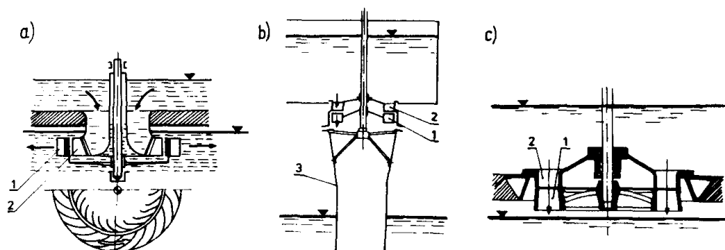
Rys. 2.4. Rozwiązania pierwszych turbin wodnych: a) turbina Foumeyrona 1827 r., b) turbina Girarda 1828 r., c) turbina Henschel-Jonval 1841-1843 r. 1 - wirnik, 2 - kierownica, 3 - dyfuzor
