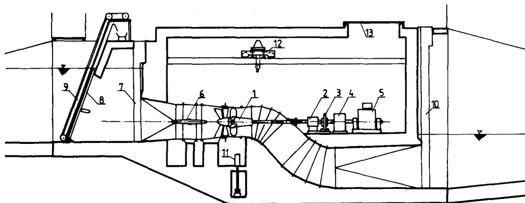
Rys. 15.10. Mała elektrownia wodna z turbiną rurową kolanową (ČKD - Blansko). 1 - wirnik turbiny z przesławnymi łopatkami, 2 - łożysko oporowe turbiny, 3 - koło zamachowe, 4 - przekładnia zębata, 5 - prądnica, 6 - zawór awaryjny motylowy (nie występuje w przypadku regulowanych łopatek kierownicy), 7 - wnęki zamknięcia remontowego wlotu, 8 - kraty wlotowe, 9 - czyszczarka krat, 10 - wnęki zamknięcia remontowego rury ssącej, 11 - agregat odwadniający, 12 - suwnica montażowa, 13 - luk nad płaszczyzną montażową
