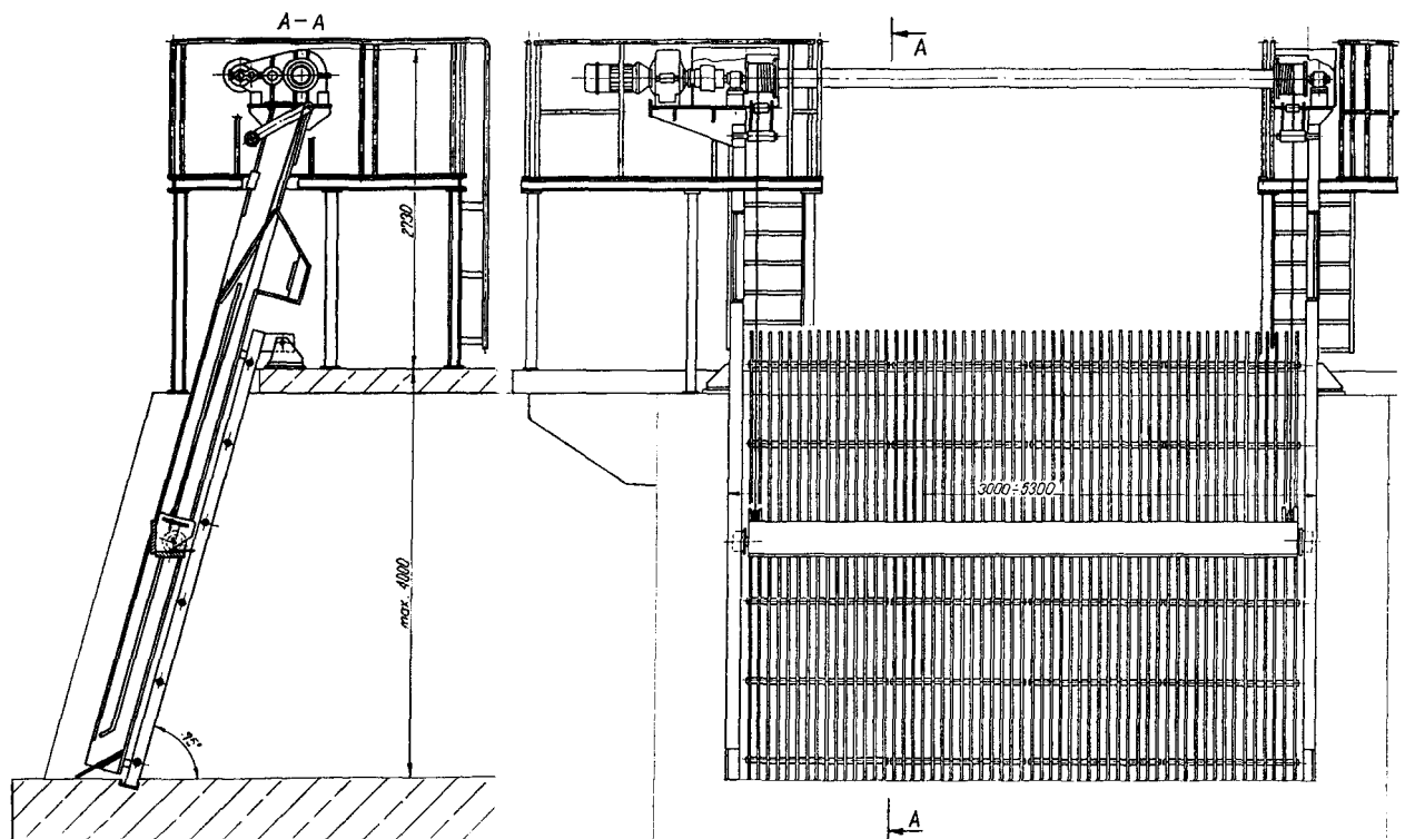
Rys. 12.2. Kraty ze stacjonarną czyszczarką
