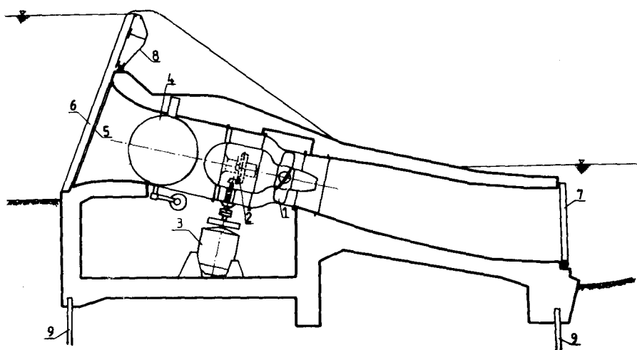
Rys. 15.8. Turbozespół z przekładnią kątową w „gruszce” (Elektrownia Rościno po przebudowie), 1 - wirnik z przestawnymi łopatkami, 2 - przekładnia zębata kątowa, 3 - prądnica z kołem zamachowym, 4 - zamknięcie awaryjne (zawór motylowy), 5 - kraty wlotowe, 6 - wnęki zamknięcia remontowego wlotu, 7 - klapowe zamknięcie remontowe rury ssącej, 8 - klapowe zamknięcie jazu
