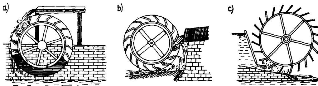
Rys. 2.2. Koła wodne o wałe poziomym: a) nasiębierne, b) śródsiębierne, c) podsiębierne
