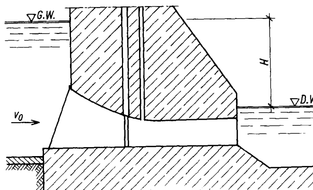
Rys. 7.8 Spust ciśnieniowy
