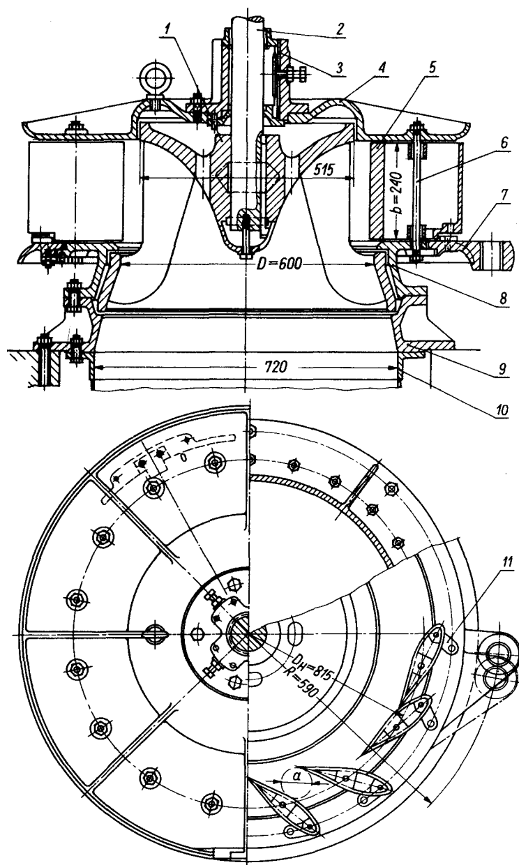
Rys. 8.10. Turbina Francisa z walem pionowym, 1 - wirnik turbiny, 2 - wał turbiny, 3 - łożysko poprzeczne (prowadzące), 4 - pokrywa kierownicy, 5 - łopatk kierownicy, 6 - sworzeń łopatki kierownicy, 7 - pierścień regulacyjny, 8 - podstawa kierownicy, 9 - pierścień podstawy, 10 - rura ssąca, 11 - łącznik
