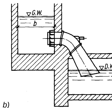
Rys. 7.17. Rura ssąca: a) z kolaniem zanurzonym w wodzie, b) z kolaniem suchym
