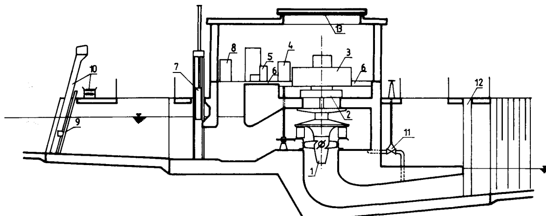
Rys. 15.6. Mała elektrownia wodna z turbiną Kaplana w komorze lewarowej (ŻRE Gdańsk - DOLMEL Wrocław), 1 - turbina Kaplana, 2 - łożysko oporowe turbozespołu, 3 - prądnica, 4 - regulator turbiny, 5 - urządzenie układu chłodzenia łożysk, 6 - kanały kablowe, 7 - zasuwa awaryjna szybkoopadająca, 8 - napęd hydrauliczny zasuwy, 9 - kraty wlotowe, 10 - czyszczarka krat, 11 - instalacja elektryczna, 12 - luk montażowy, 13 - wnęki zamknięcia remontowego rury ssącej, 17 - luk montażowy
