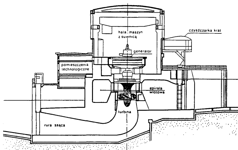
Rys. 8.14. Elektrownia z pionową turbiną Kapłana zabudowana w komorze spiralnej
