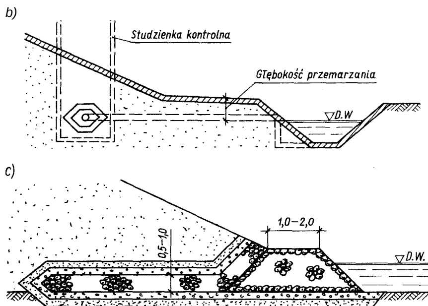
Rys. 7.5. Drenaż stopy skarpy odpowietrznej zapory: a) przyzma drenażowa, b) drenaż rurowy, c) drenaż piaski wewnętrzny
