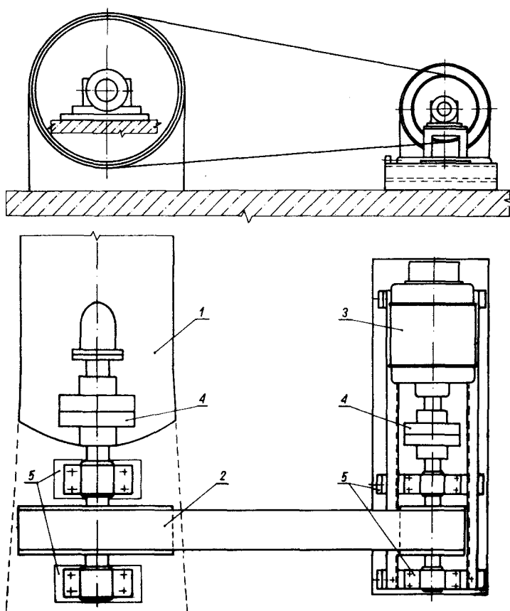
Rys. 10.7. Przekazanie napędu z turbiny na prądnicę za pomocą przekładni z pasami klinowymi w układzie pionowym wałów turbiny i prądnicy, 1 - wał turbiny, 2 - przekładnia, 3 – prądnica
