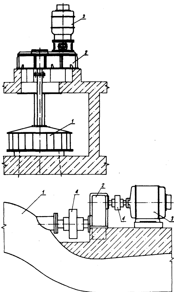
Rys. 10.5. Przekazanie napędu z turbiny na prądnicę za pomocą przekładni zębatej walcowej poziomej, 1 - turbina rurowa, 2 - przekładnia, 3 - prądnica, 4 - sprzęgło
