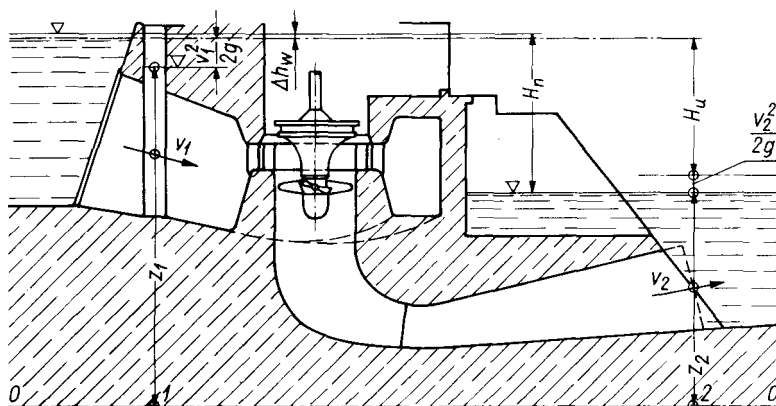
Rys. 8.2. Spad niwelacyjny H_n i użyteczny H_u turbiny oraz straty wlotowe h_{w1} . Ogólnie spad użyteczny określa się więc
