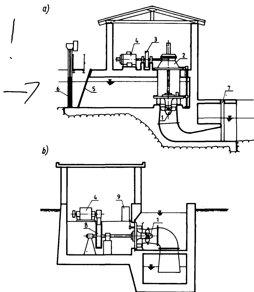
Rys. 15.5. Rozwiązanie MEW z turbinami Kaplana w komorach otwartych (ČKD Blansko): a) z turbiną pionową, b) z turbiną poziomą, 1 - turbina Kaplana, 2 - przekładnia kątowna zębata, 3 - koło zamachowe, 4 - prądnica, 5 - kraty wlotowe, 6 - zamknięcie remontowo-awaryjne, 7 - wneki zamknięcia remontowego rury ssącej, 8 - przekładnia pasowa, 9 - regulator turbiny
