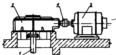
Rys. 10.4. Przekazanie napędu z turbiny na prądnicę za pomocą przekładni zębatej stożkowej. 1 - wał turbiny, 2 - przekładnia, 3 - prądnica, 4 - sprzęgło
