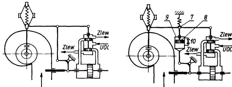
Rys. 9.2. Regulator obrotów z dużym statyzmem regulacji
