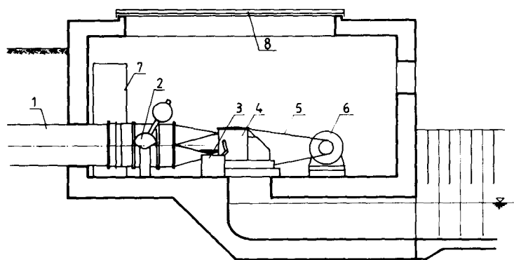
Rys. 15.12. Rozwiązanie MEW z turbiną Banki (ŻRE Gdańsk), 1 - rurociąg doprowadzający, 2 - zawór motylowy z zamknięciem ciężarowym, 3 - regulator turbiny, 4 - turбина Banki, 5 - pas transmisyjny, 6 - prądnica, 7 - szafa sterowniczo-rozdzielcza, 8 - luk montażowy
