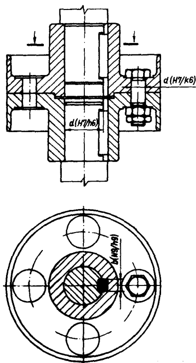
Rys. 10.1 Sprzęgło sztywne
